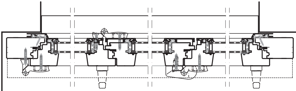
Horizontalschnitt Massstab 1:5
