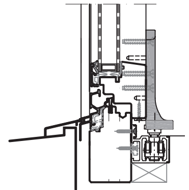
Vertikalschnitt oben und unten Massstab 1:5
