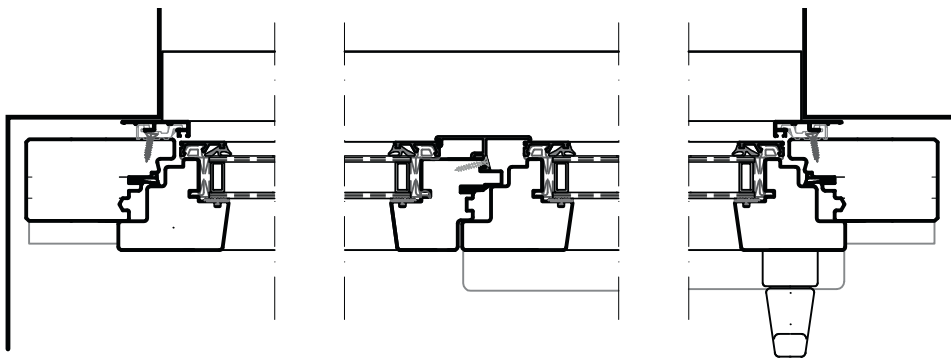
Horizontalschnitt Massstab 1:5
