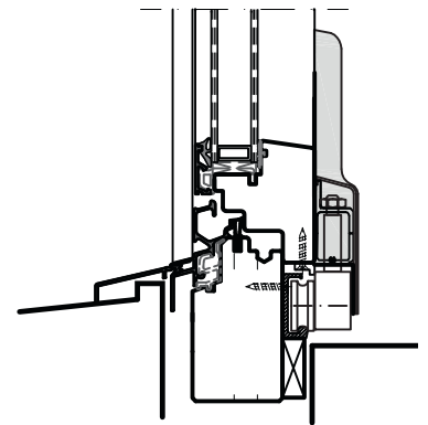
Vertikalschnitt oben und unten Massstab 1:5
