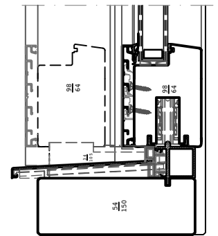
Vertikalschnitt oben und unten Massstab 1:5
