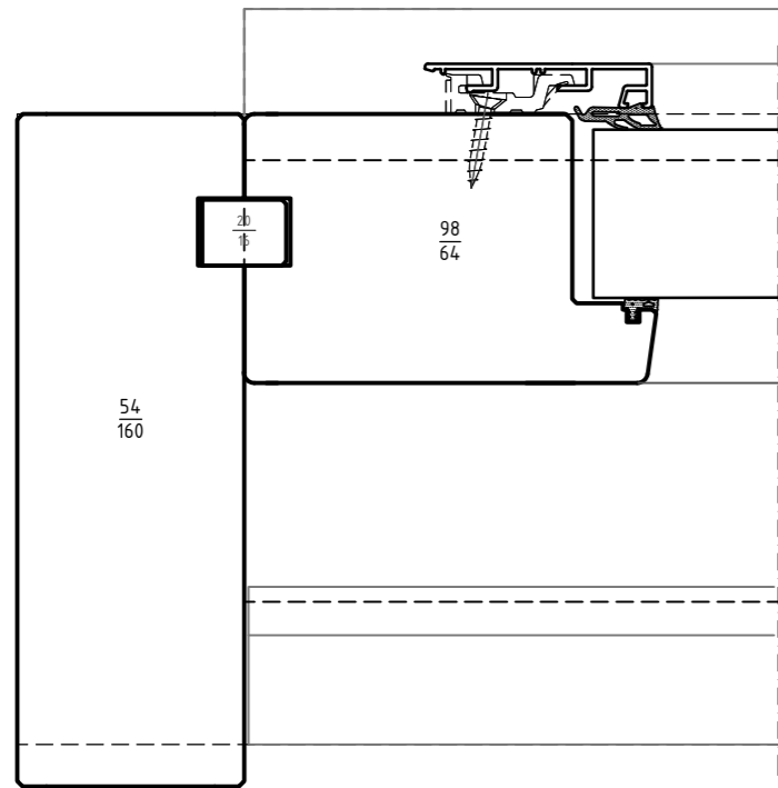
Horizontalschnitt Abschluss links
