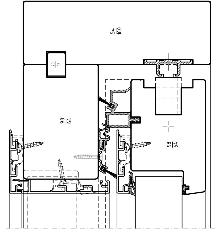
Vertikalschnitt Abschluss oben
