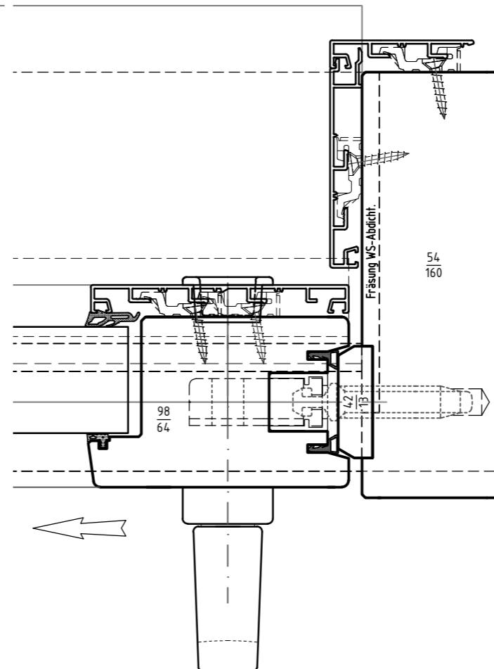
Horizontalschnitt Abschluss rechts
